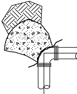
90° BEND
