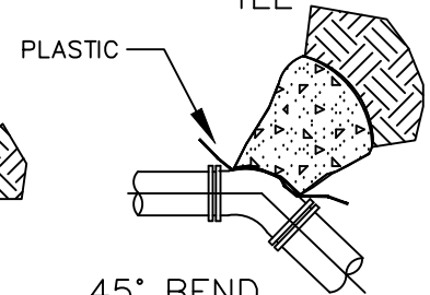
45° BEND
